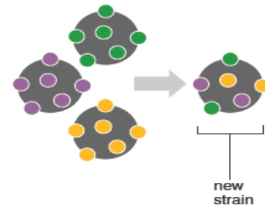
Antigenic shift
